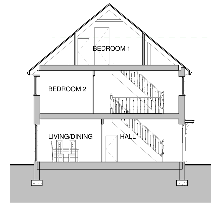
Section A 1 : 100
